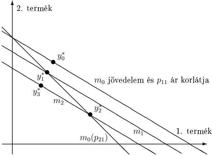
1. ábra. A Giffen-hatás elemzése két változó esetén
