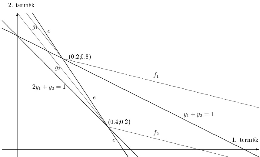
2. ábra. A (0.2; 0.8) ponton átmenő közömbösségi görbe két ága f_1 és g_1 , míg a (0.4; 0.2) ponton átmenő közömbösségi görbe két ága f_2 és g_2 .
