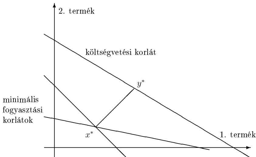
3. ábra. Az optimális megoldáspár egy kötelező minimális fogyasztású modellben
